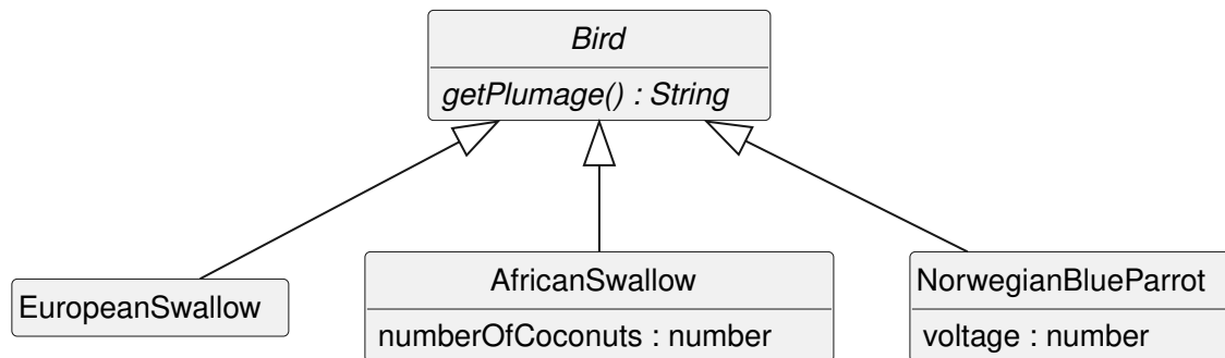
FIGURE 6.3. – Classes « Bird » auxquelles on a appliqué le principe GRASP Polymorphisme. (PlantUML)
