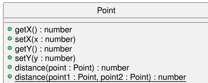
FIGURE 5.1. – Les méthodes publiques d’une classe sont un exemple d’interface API. (PlantUML)
