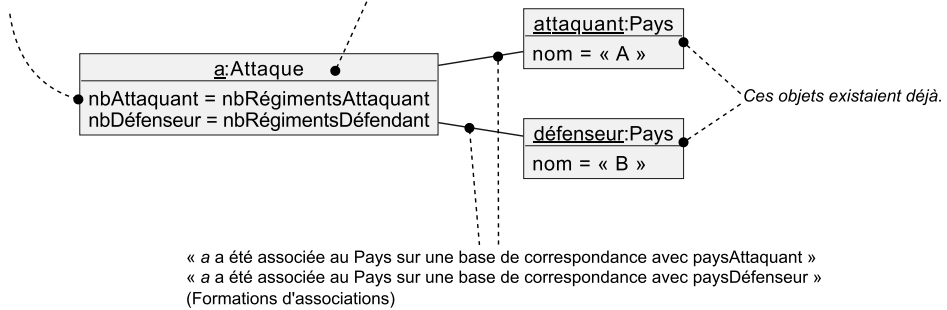
FIGURE 8.2. – Les postconditions décrivent la manipulation d'objets dans un MDD (la partie inférieure ici est un diagramme d'objets).
