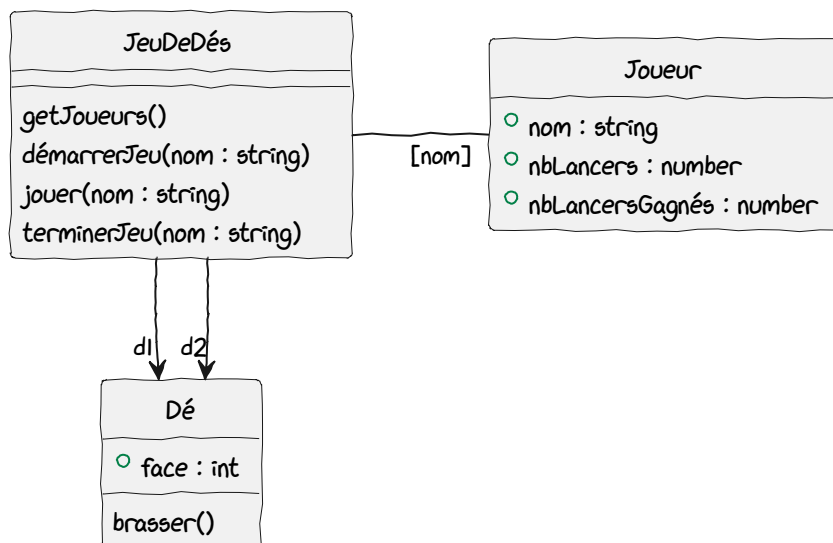
FIGURE 1.2. – Diagramme de classes logicielles décrivant une solution au problème du jeu de dés. La conception s'inspire du modèle du problème, afin de faciliter sa compréhension. (PlantUML)
