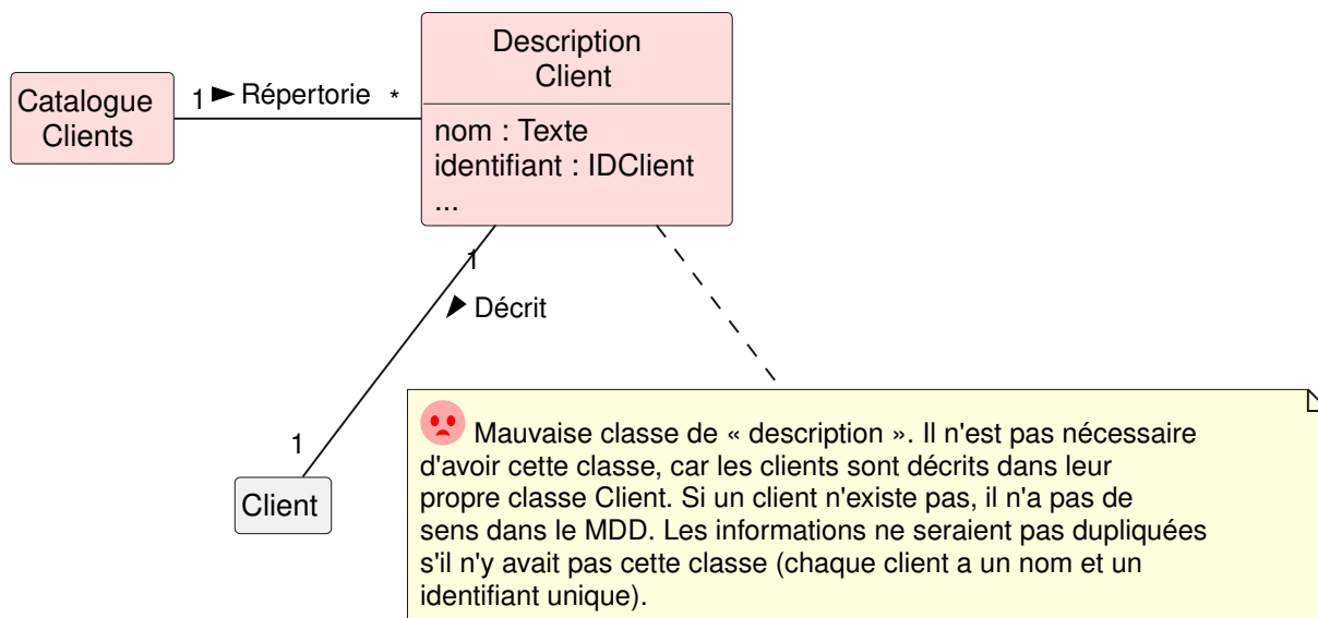
FIGURE 4.4. – Illustration d’une erreur fréquente : utiliser une classe de description sans justification. (PlantUML)
