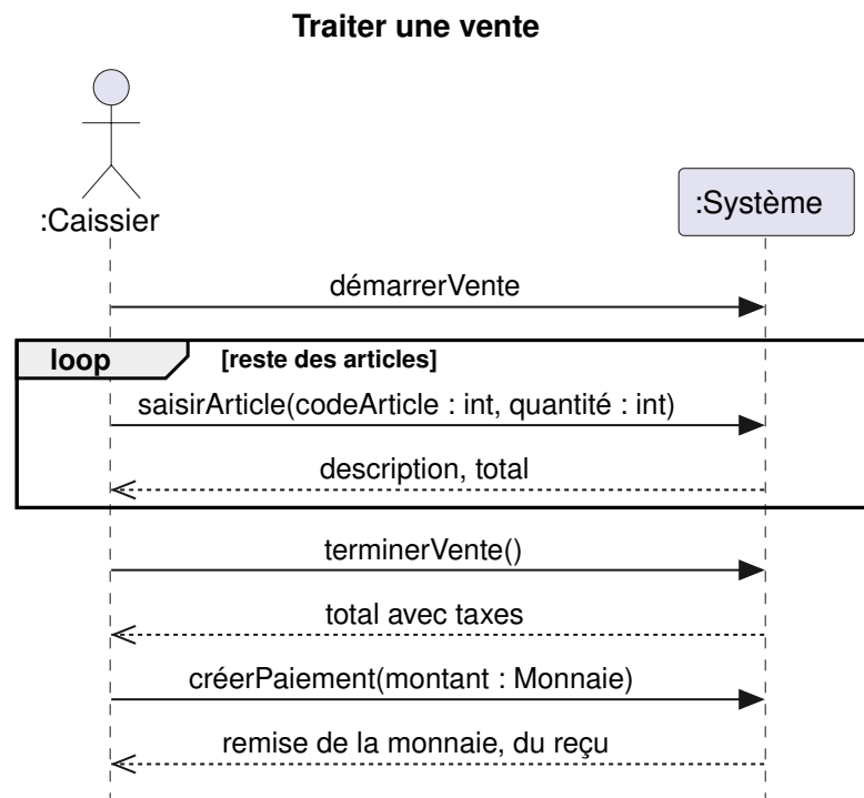
FIGURE B.1. – DSS pour le scénario Traiter une vente de Larman (2005). (PlantUML)
