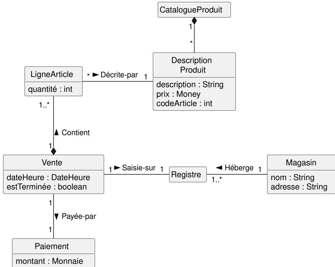
FIGURE B.2. – MDD pour le scénario Traiter une vente de Larman (2005). (PlantUML)
