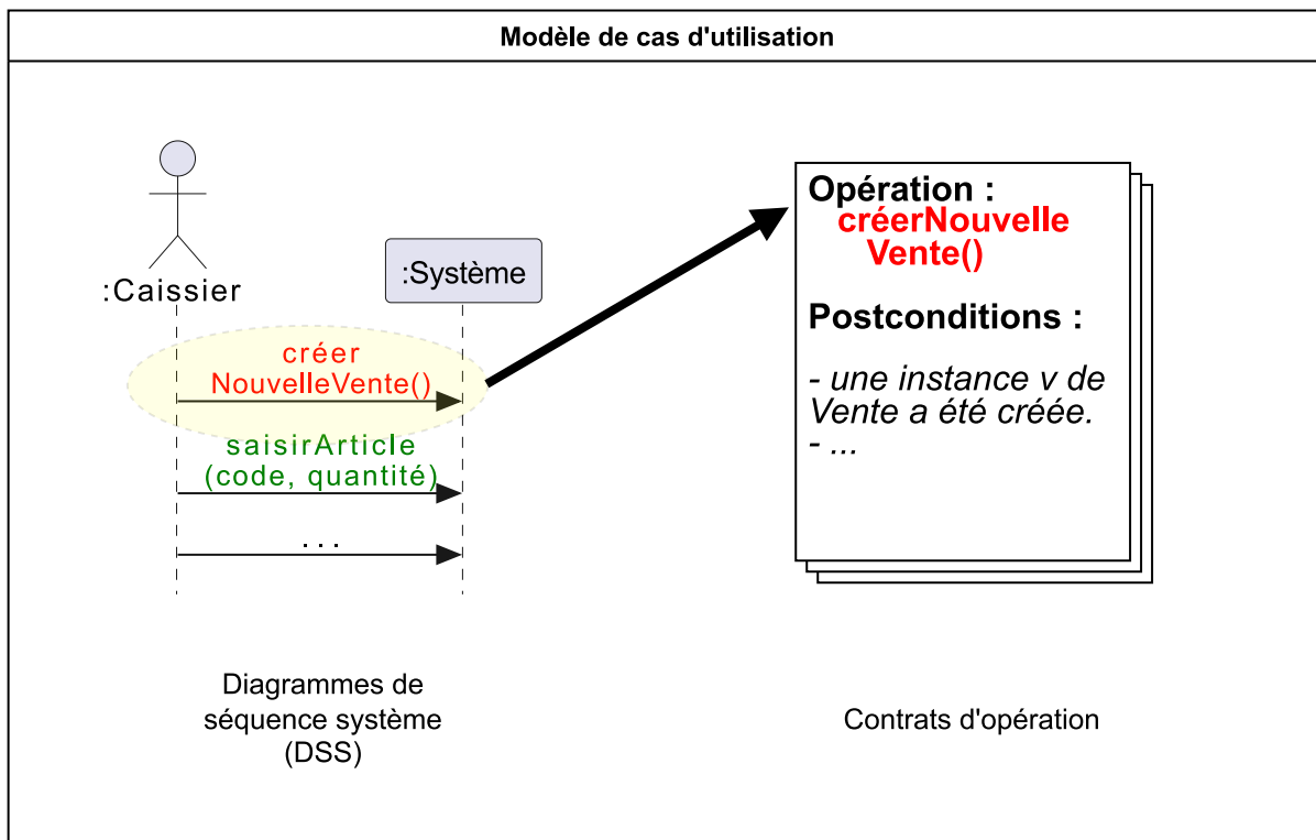
FIGURE 8.1. – Pendant l'opération système créerNouvelleVente , une instance de Vente doit être créée. Le contrat d'opération le spécifie dans une postcondition : une instance v de Vente a été créée.
