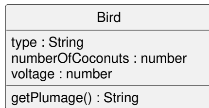
FIGURE 6.2. – Classe « Bird » à laquelle on peut appliquer le principe GRASP Polymorphisme. (PlantUML)
