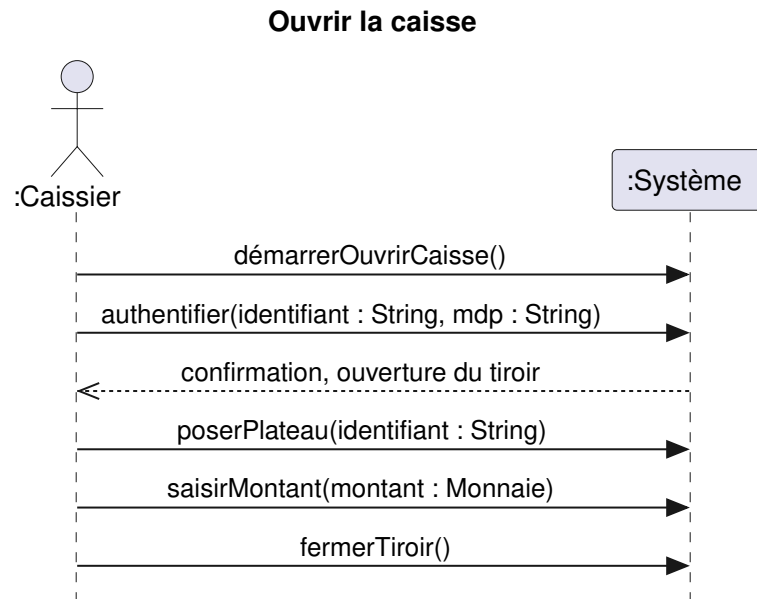
FIGURE C.3. – Diagramme de séquence système (DSS) pour le scénario Ouvrir la caisse . (PlantUML)
