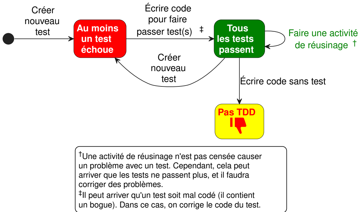
FIGURE 10.1. – États du développement piloté par les tests. (PlantUML)
