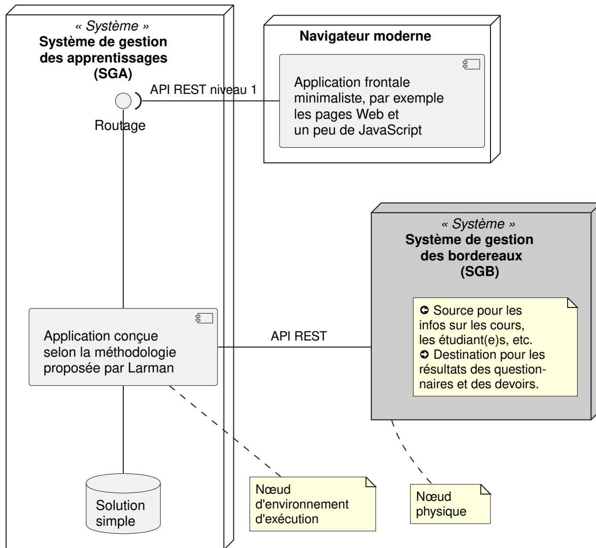
FIGURE 19.1. – Diagramme de déploiement du système à développer pour le laboratoire. (Plan-tUML)
