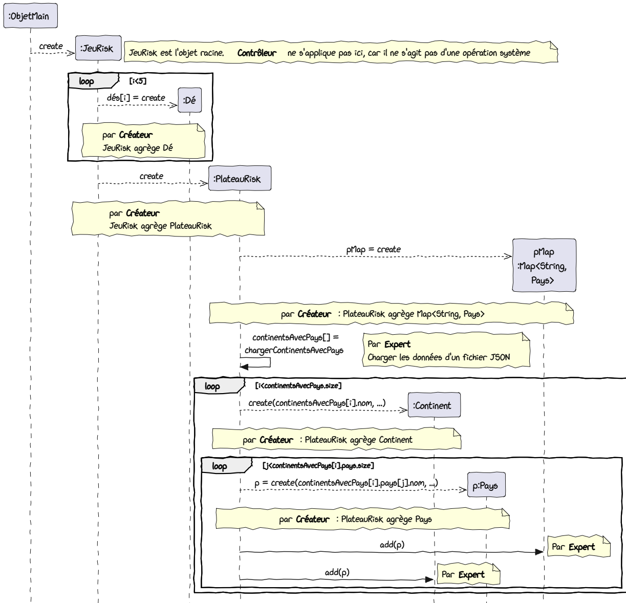
FIGURE 9.6. – Exemple de l'initialisation partielle du jeu Risk, avec les principes GRASP et les tableaux associatifs pour faciliter la transformation d'identifiants en objets. (PlantUML)
