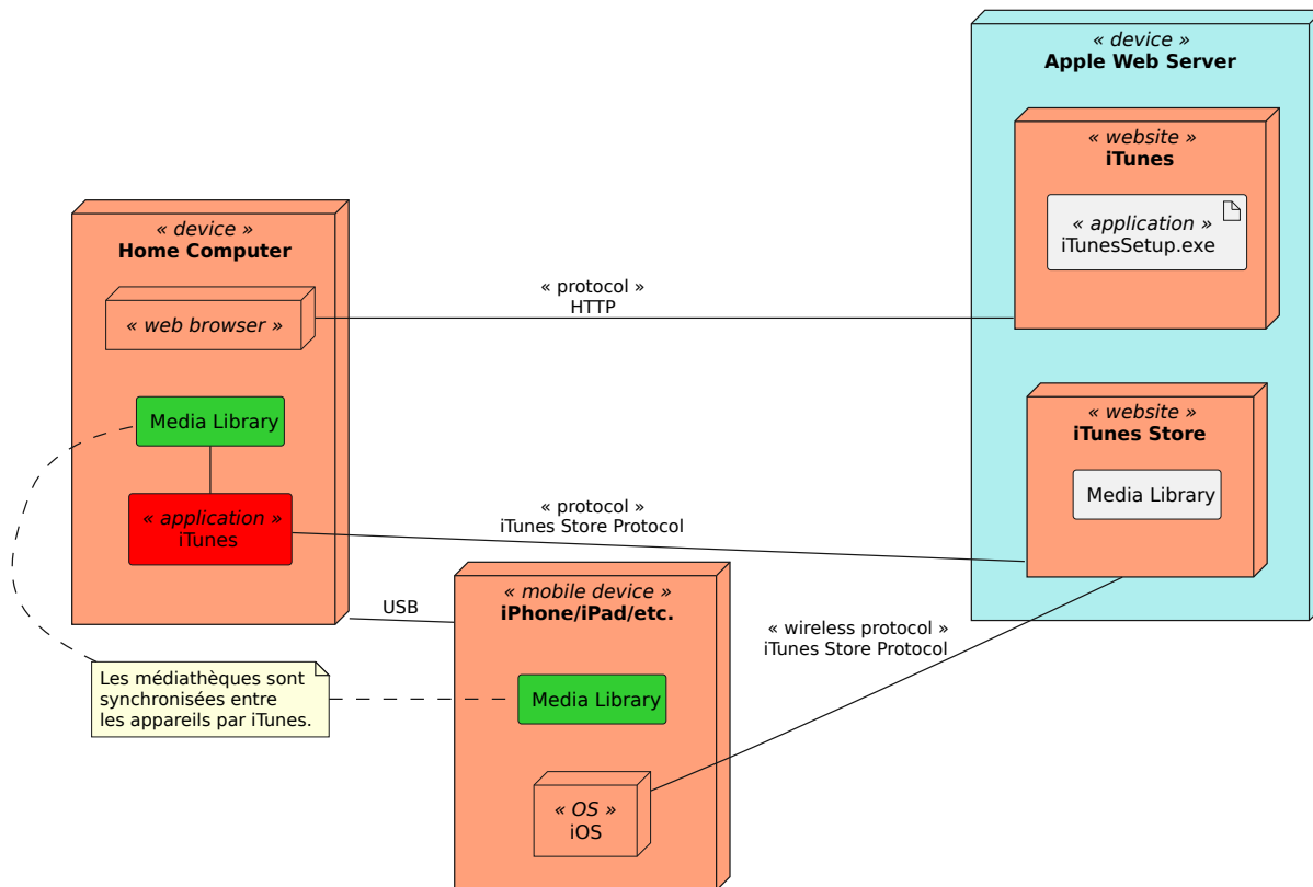
FIGURE 19.2. – Diagramme de déploiement pour iTunes d’Apple avec un ordinateur, un iPad et le service Web d’Apple, selon ce modèle UML de Kirill Fakhroutdinov (utilisé avec permission). (PlantUML)
