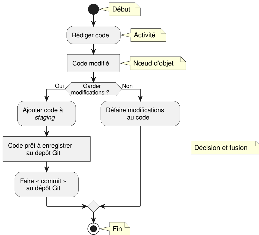
FIGURE 16.1. – Diagramme d'activité pour un processus simple avec Git. (PlantUML)
