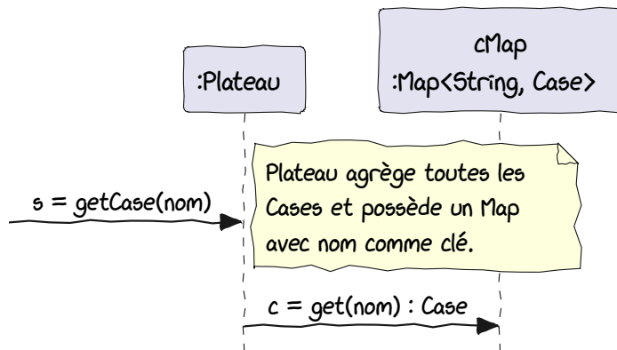
FIGURE 9.5. – Exemple de l'utilisation d'un tableau associatif pour trouver une Case Monopoly à partir de son nom. (PlantUML)
