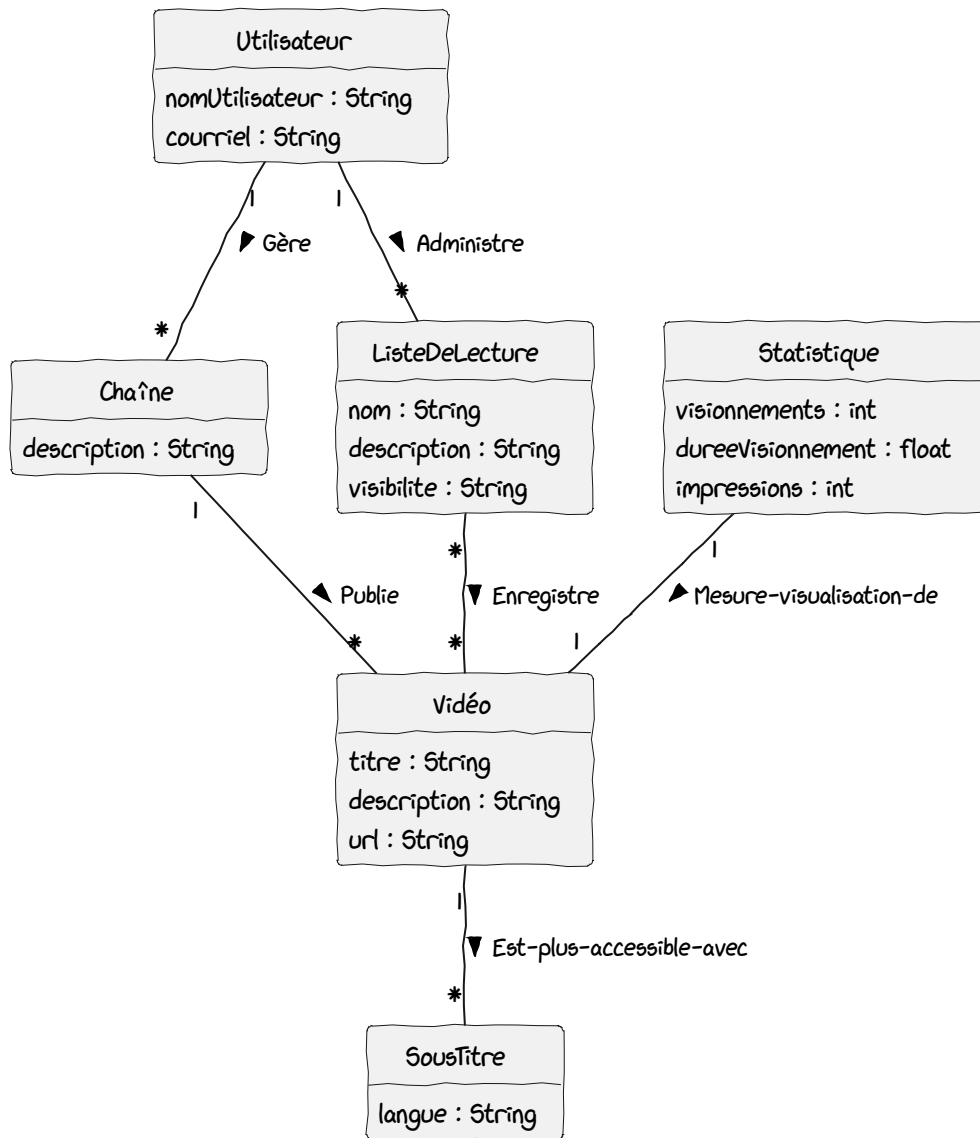
FIGURE 4.9. – Modèle du domaine partiel pour le logiciel YouTube avec des verbes d’association plus riches. (PlantUML)
