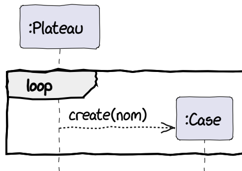
FIGURE 9.2. – Combiner la création d'une instance et une modification de son attribut dans un constructeur. (PlantUML)
