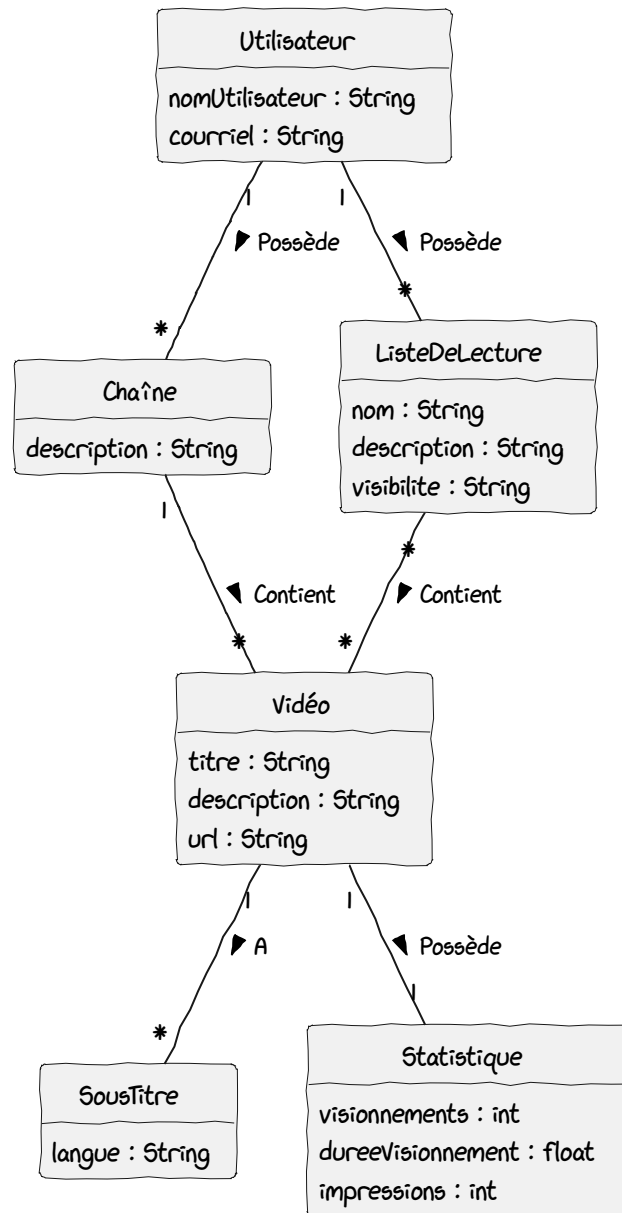
FIGURE 4.8. – Modèle du domaine partiel pour le logiciel YouTube. (PlantUML)
