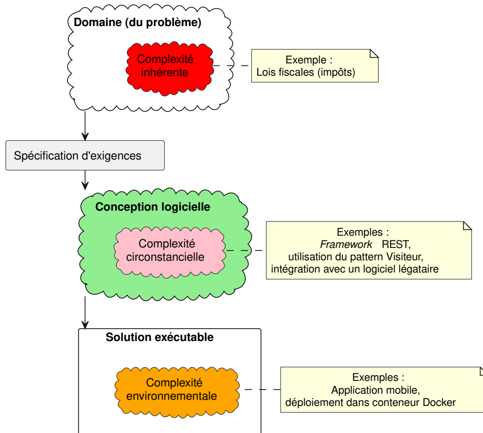
FIGURE 1.4. – Sources de complexité (inhérente, circonstancielle et environnementale) par rapport au processus de développement (analyse, conception et implémentation). (PlantUML)
