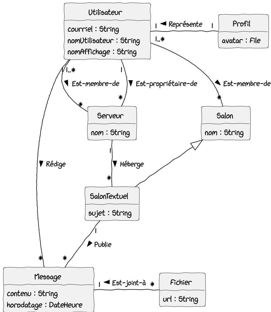
FIGURE 4.7. – Associations et cardinalités des classes conceptuelles proposées dans l'exercice. (PlantUML)
