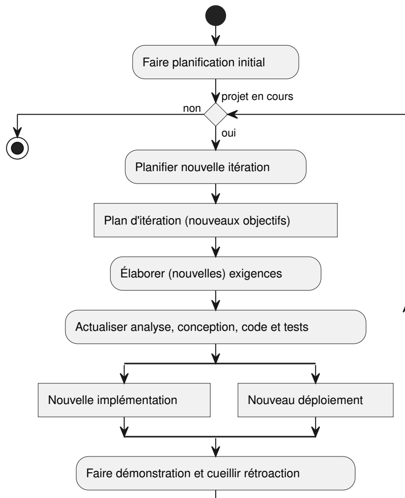
FIGURE 1.6. – Un processus itératif permet de gérer les complexités, car la planification d'une itération peut viser une partie du système et le système évolue à mesure que les itérations avancent. (PlantUML)
