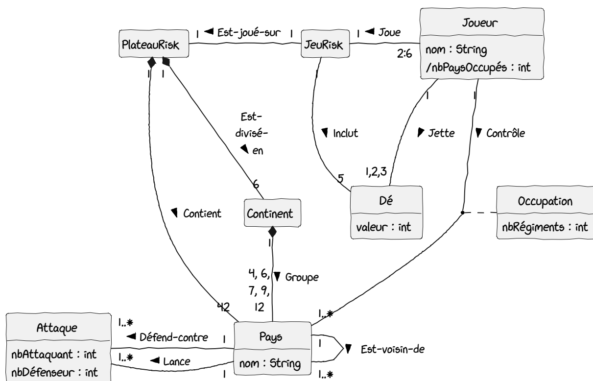
FIGURE 4.2. – Modèle du domaine du jeu Risk. (PlantUML)
