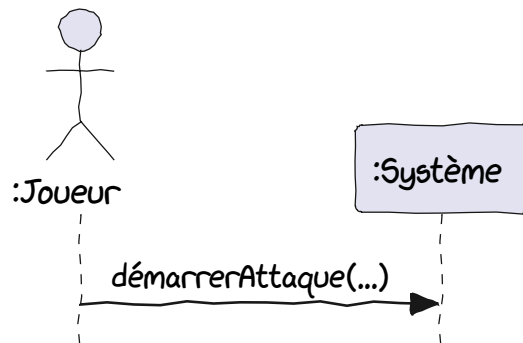
FIGURE 5.6. – Une opération système dans un DSS. C'est une abstraction. (PlantUML)
