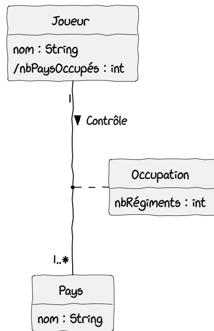
FIGURE 4.5. – Classe d’association dans le MDD Jeu Risk. (PlantUML)
