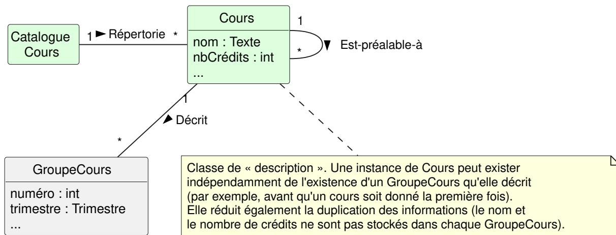
FIGURE 4.3. – La classe Cours joue le rôle de description d'entités (les groupes-cours). (PlantUML)
