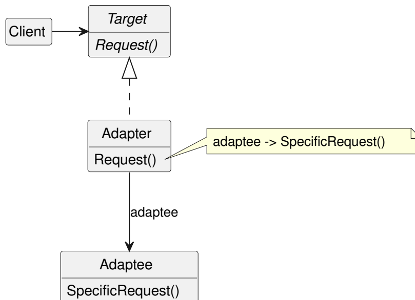
FIGURE 14.1. – Le diagramme de classes du pattern Adaptateur (Gamma et coll., 1994). (PlantUML)
