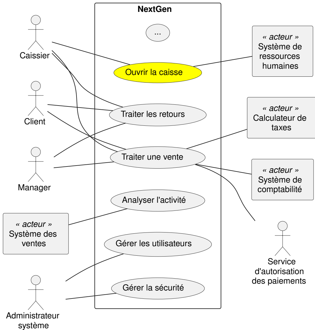
FIGURE C.1. – Diagramme de cas d'utilisation pour le système NextGen. (PlantUML)
