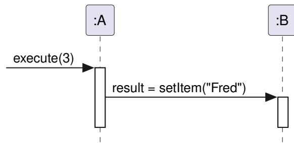
FIGURE 9.8. – Exemple de diagramme de séquence. (PlantUML)
