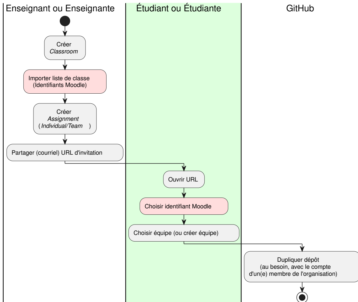
FIGURE 16.2. – Diagramme d'activités pour les activités séquentielles de GitHub Classroom (contexte de l'ÉTS avec Moodle). (PlantUML)
