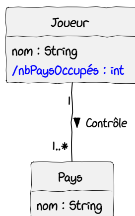
FIGURE 4.1. – nbPaysOccupés est un attribut dérivé. Sa valeur sera calculée selon le nombre de pays de l'association. (PlantUML)
