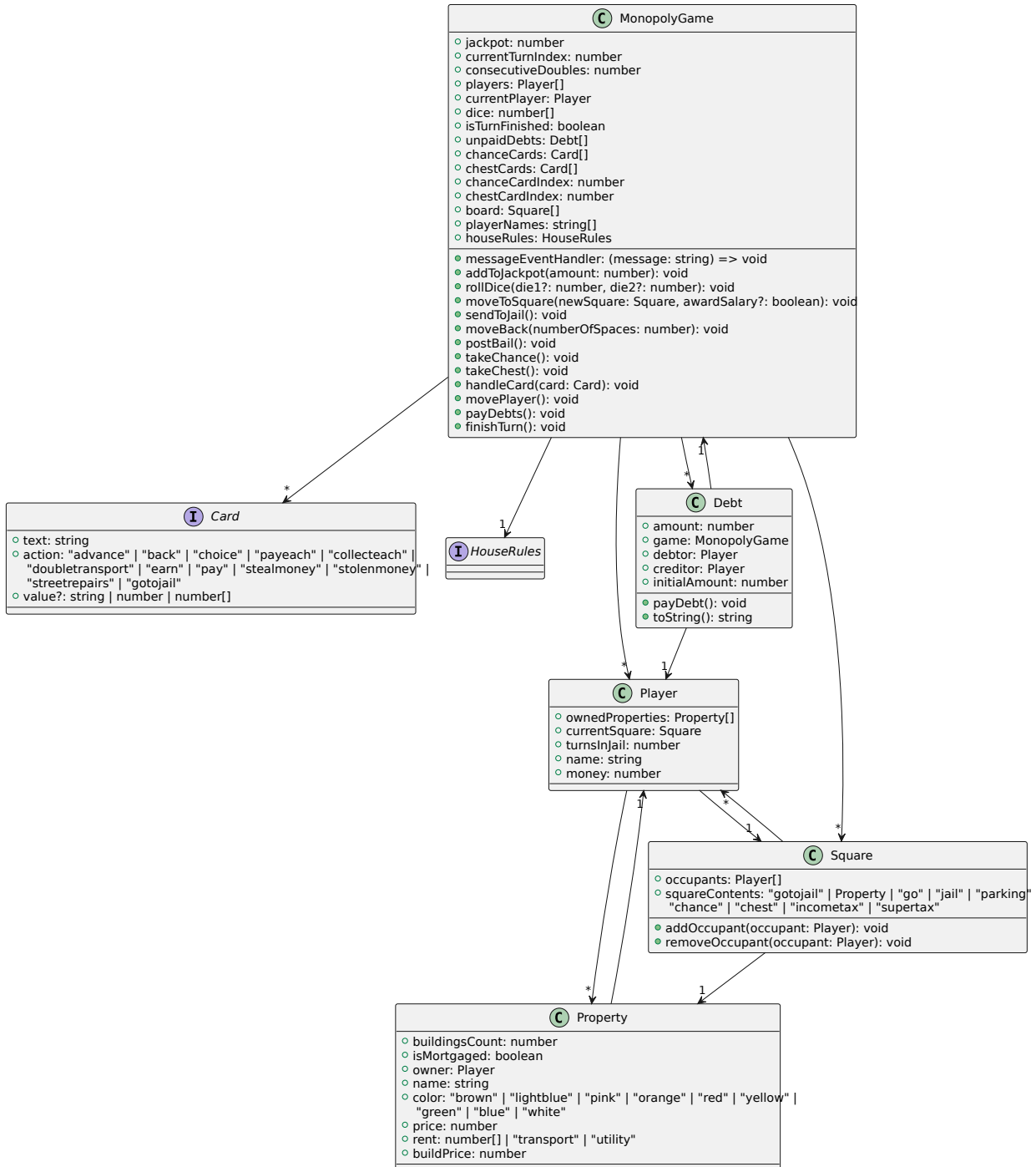
FIGURE 9.9. – Diagramme de classes logicielles (TypeScript) pour le projet Emojiopoly . (PlantUML)
