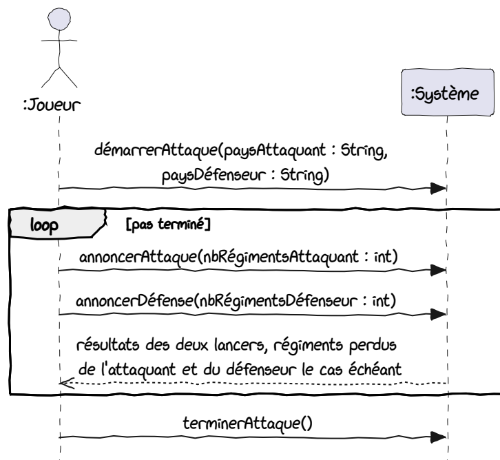
FIGURE 5.5. – Diagramme de séquence système pour le scénario Attaquer un pays . (PlantUML)
